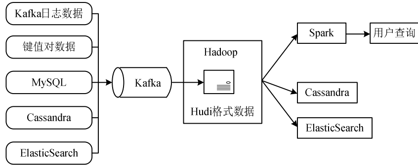
图 22.4 Kappa+架构
