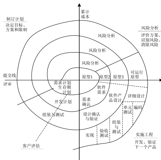
图 7.4 螺旋模型
